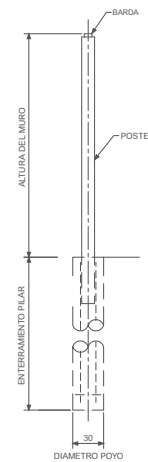
SECCION - DEL MURO Y PILAR
