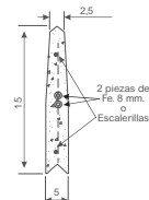
SECCION - PLACA REFORZADA
