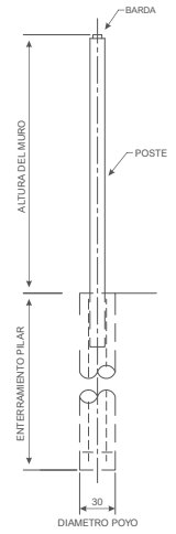
SECCION - DEL MURO Y PILAR
