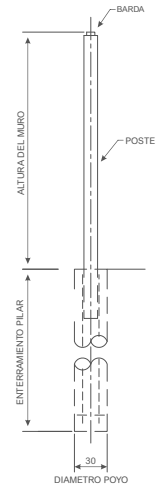
SECCION - DEL MURO Y PILAR
