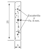
SECCION - PLACA
