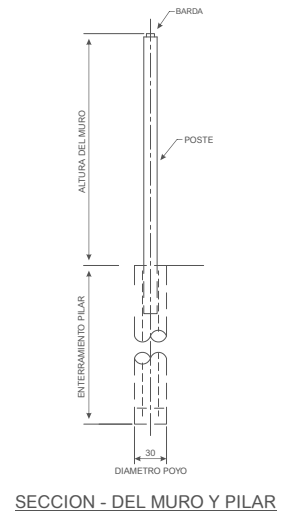
SECCION - DEL MURO Y PILAR
