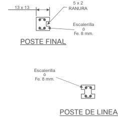
SECCION - DEL PILAR
