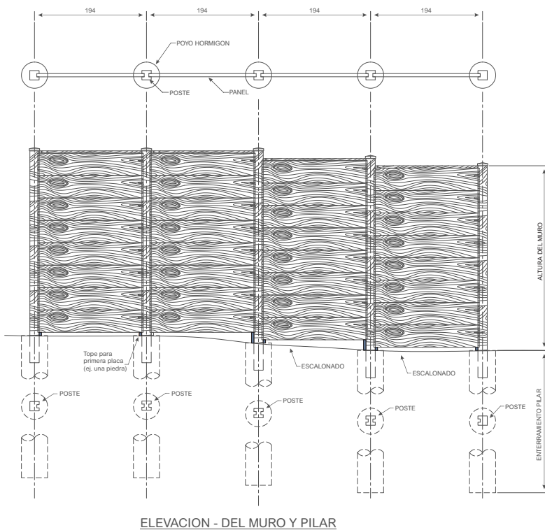
ELEVACION - DEL MURO Y PILAR
