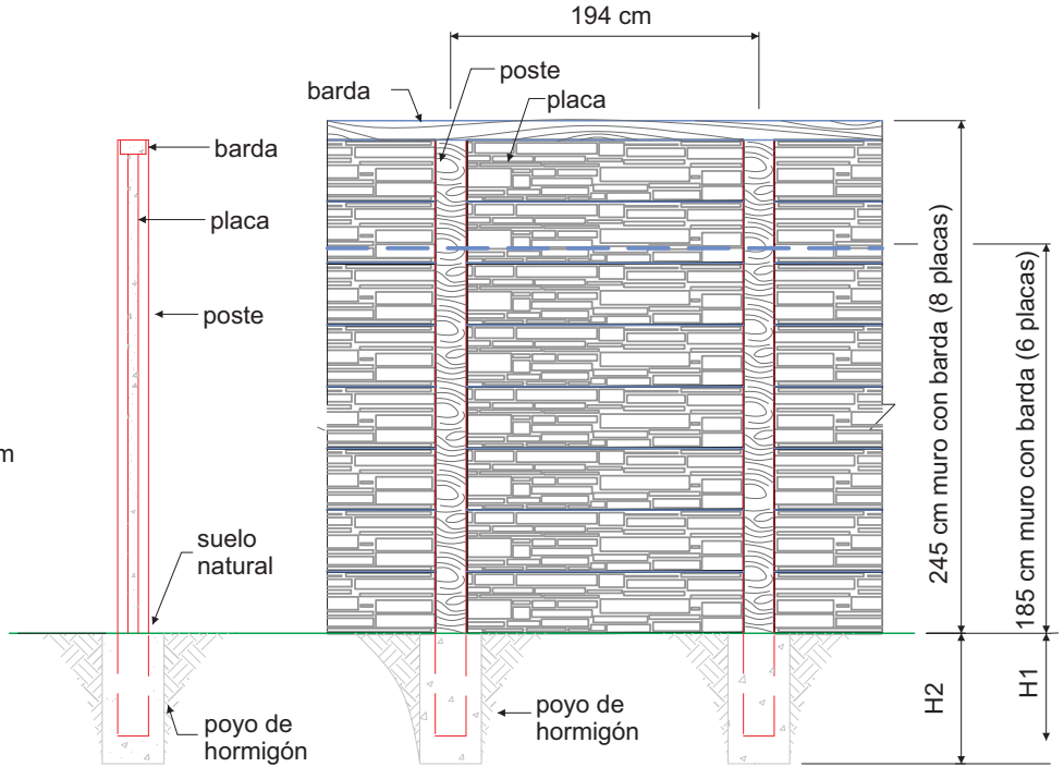
MURO PIEDRA - SECCION
